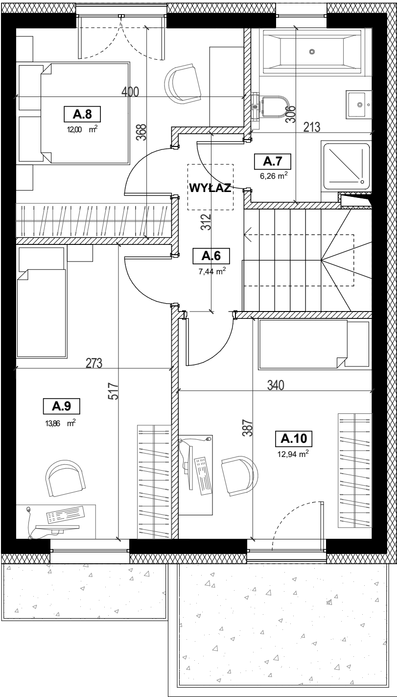
RZUT PIĘTRA
